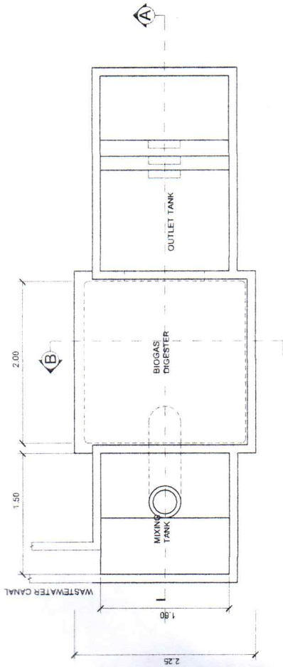
PLAN SCALE 1:50 M.
