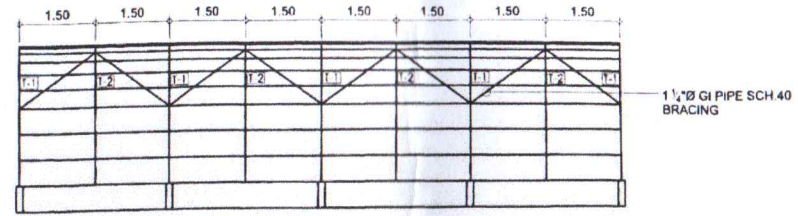
LONGITUDINAL SECTION SCALE 1:100 M.
