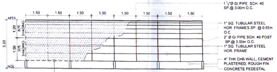
TYP. SIDE ELEVATION SCALE 1:100 M.
