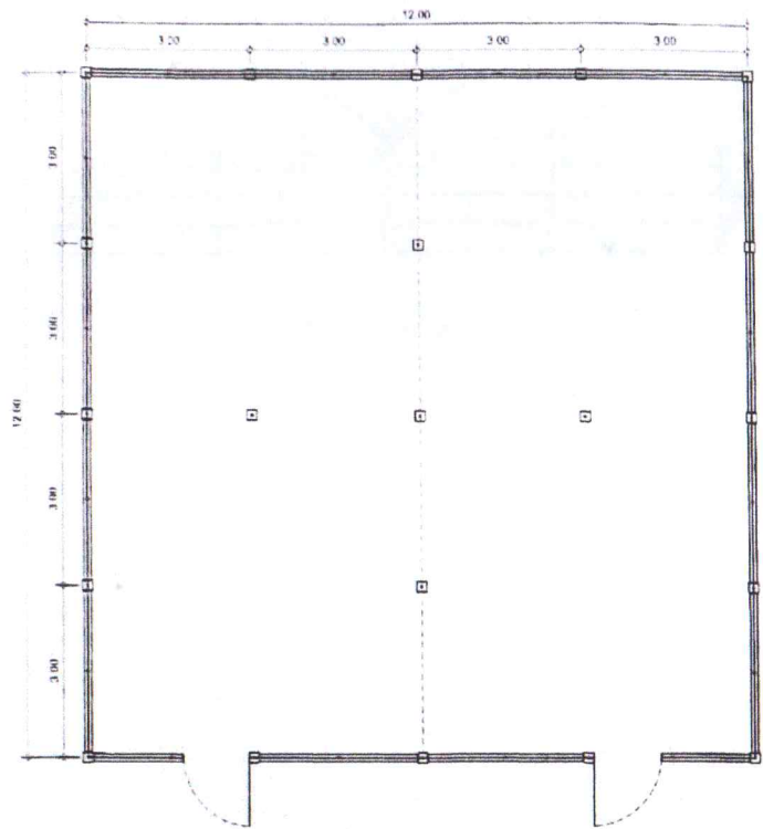
P L A N SCALE 1:100 M.
