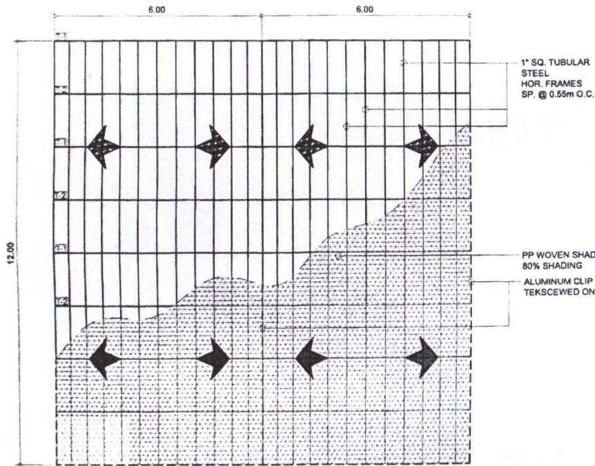
TOP ELEVATION SCALE 1:100 M.
