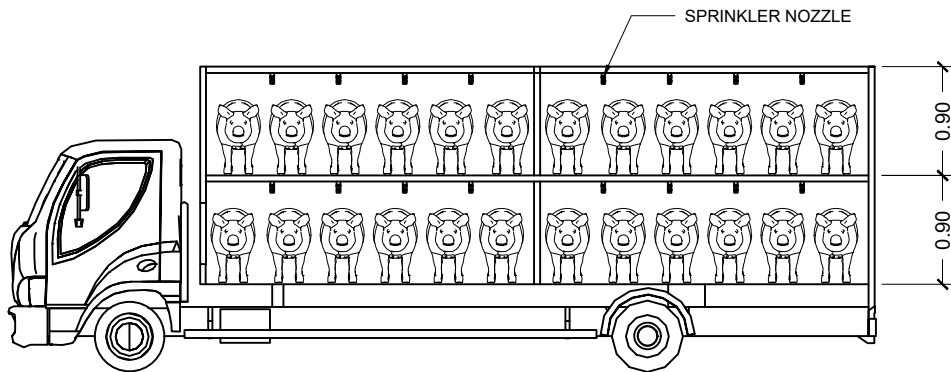
LONGITUDINAL SECTION THRU "A-A" Scale: NTS
