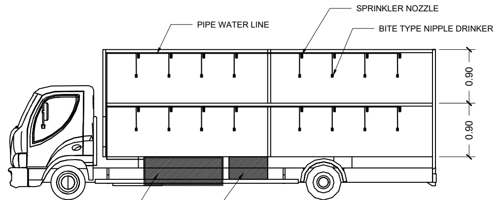
SECTION THRU "X-X" Scale: NTS
