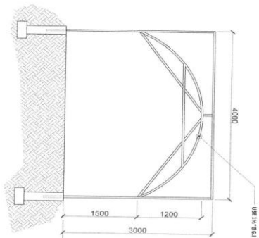
A FRONT ELEVATION SCALE: 1:70
